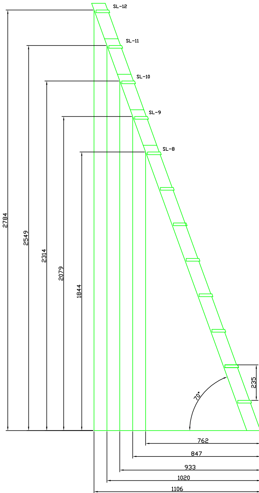
SL Stufenleiter mit Buchestufen Fa. Weiblen Spezialwerkzeuge
